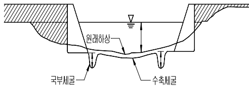
수축세굴과 국부세굴
