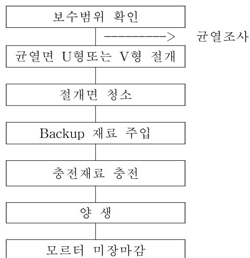
<그림 4.2.7> 철근이 부식하지 않는 경우의 충전공법 및 시공흐름
