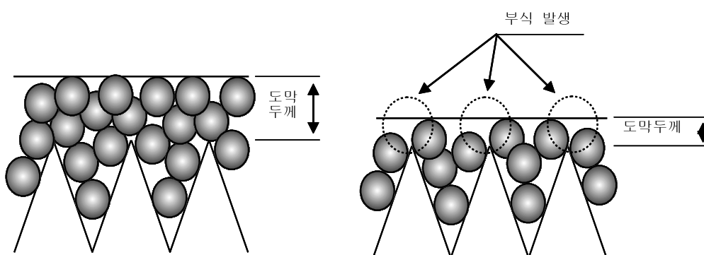
(a) 정상적인 도막두께
