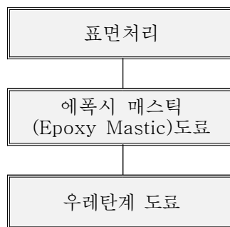
<그림 4.2.13> 보수도장 방법 개요도(재도장하는 경우)
